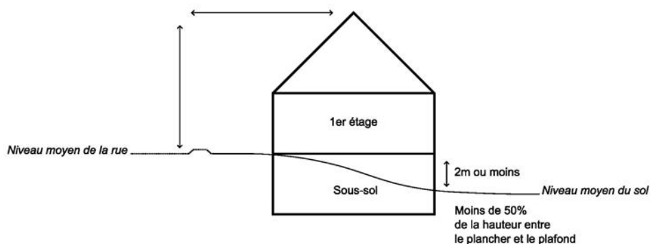
Croquis 16 : Étage
